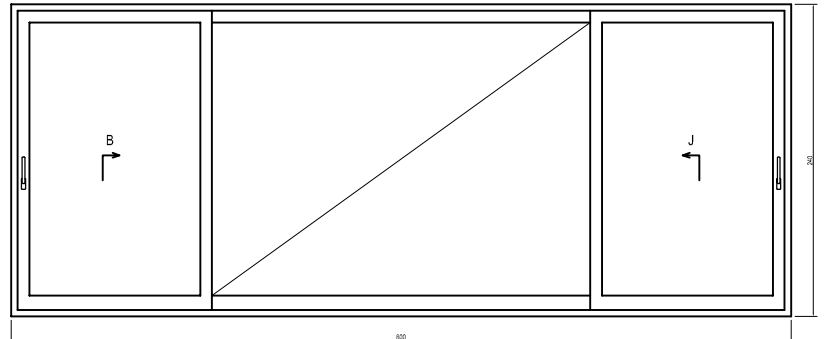
"K" séma 2 emelő-toló mozgó szárny, 1 fix szárny
