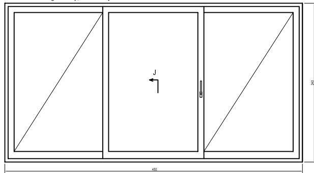
"G" séma 1 emelő-toló mozgó szárny, 2 fix szárny
