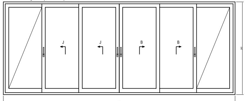
"L" séma 4 emelő-toló mozgó szárny, 2 fix szárny
