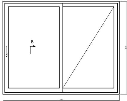
"A" séma 1 emelő-toló mozgó szárny, 1 fix szárny
